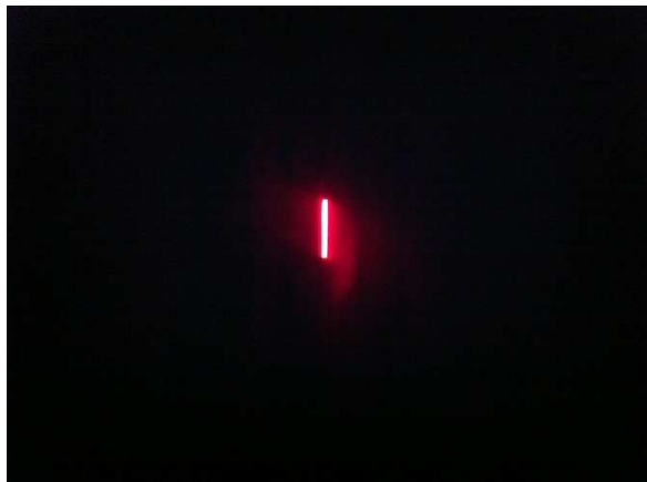
656nm (Halpha)
