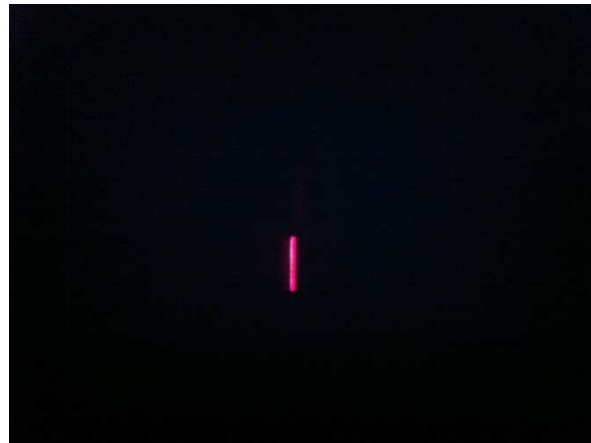
673nm ([SII])
